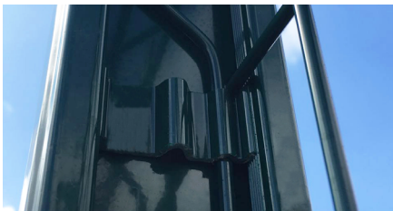
CLIP FIXATION POTEAU/PANNEAU Vis 6x40 + écrou autocassant
